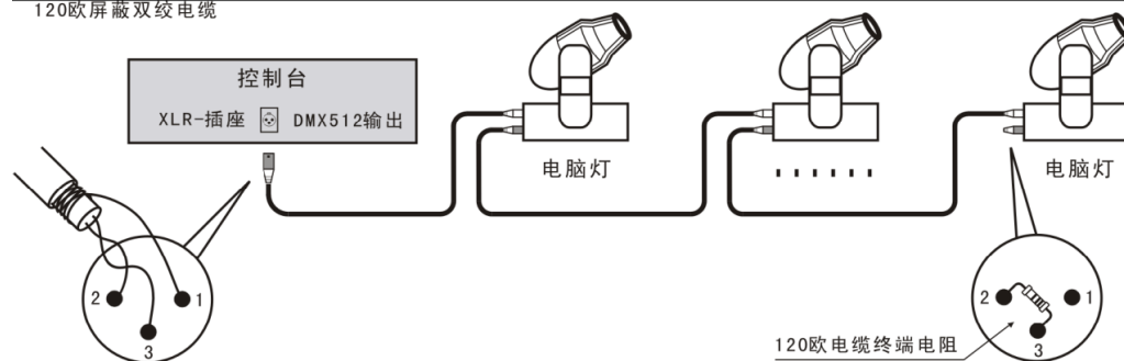
120欧屏蔽双绞电缆
